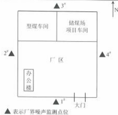
图 4-6 厂界噪声监测点位示意图
