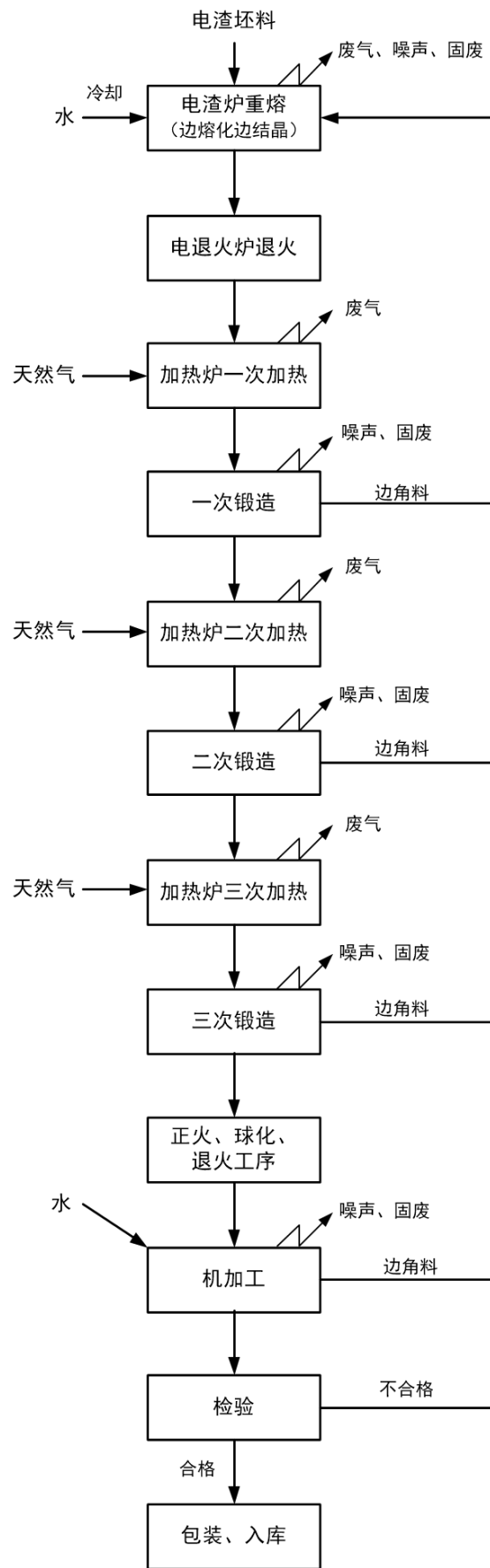
冷轧辊生产工艺流程及产污节点图
